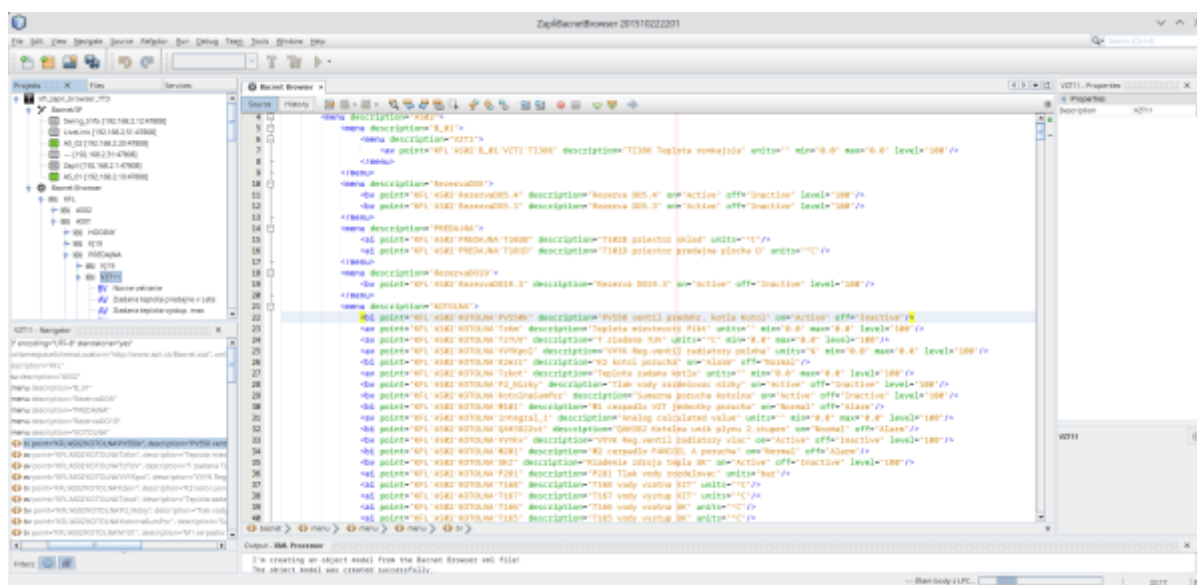
Webové rozhranie
